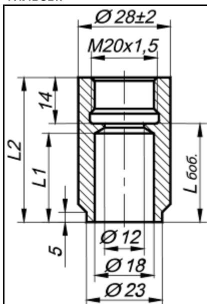
Рис. 1 Бобышка прямая БПТ-01-М20х1,5-L
